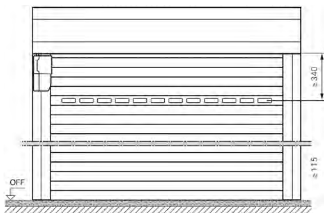
Einbau hinten / in der Öffnung - Innen-Rollltor
