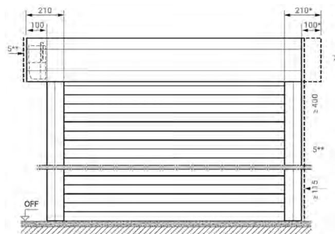
Einbau vor der Öffnung - Außen-Rollltor
