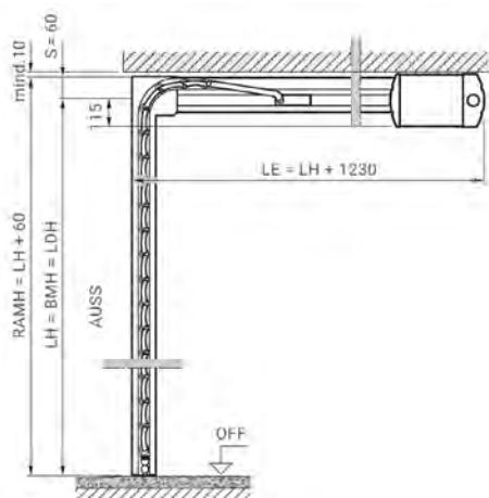
Einbau in der Öffnung, Ansicht innen
